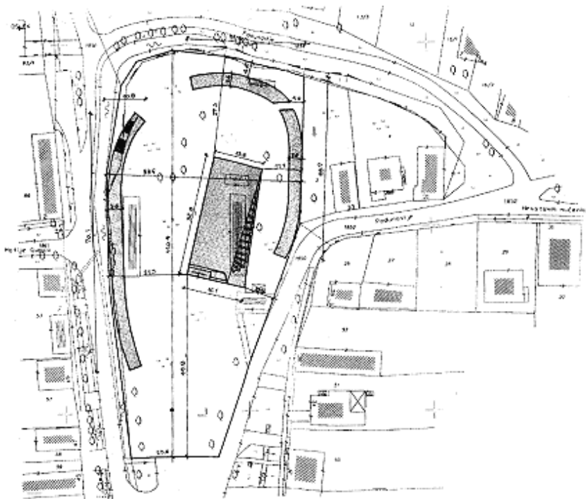
Situacija gradilišta na izvodu iz katastarskog plana
