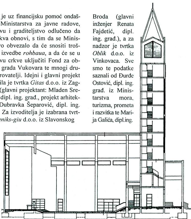
Uzdužni presjek kroz novu crkvu
