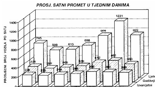
Slika 7. Kolebanje prometa po danima u tjednu na lokaciji Jošan za različita razdoblja promatranja [1]
