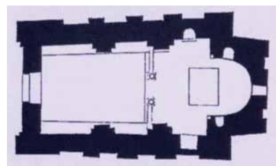
Tlocrt crkve Sv. Ivana Krstitelja (T. Marasović)
