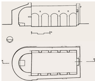
Presjek i tlocrt crkve Sv. Ivana
