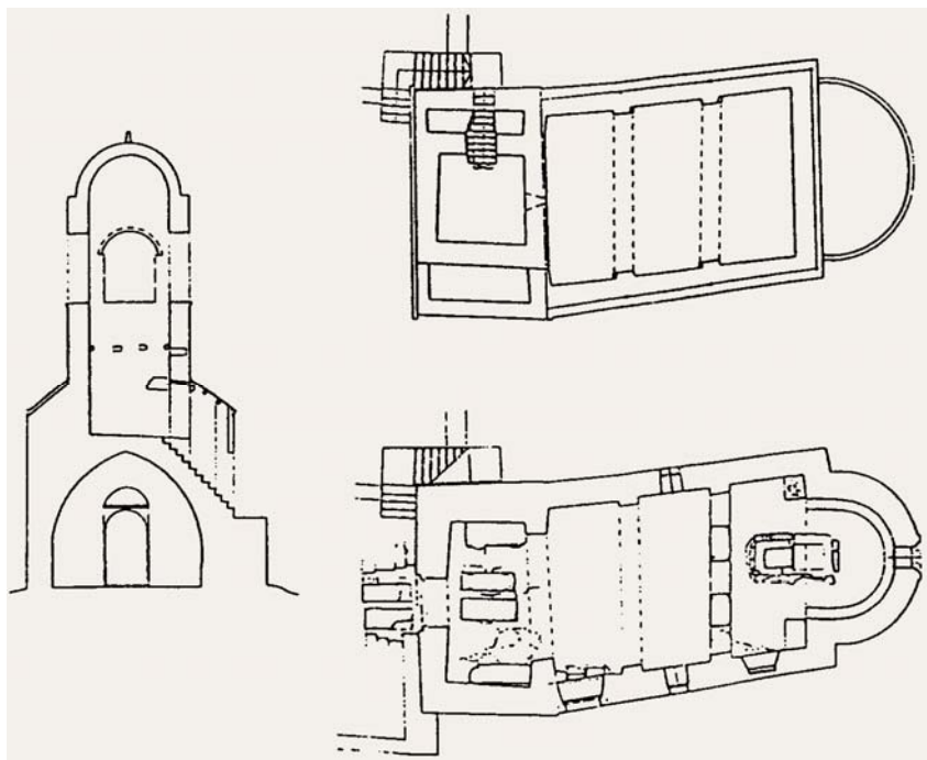
Snimak stanja i arheoloških istraživanja crkve Gospe od Lužine (N. Nad)
