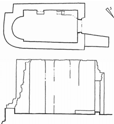
Tlocrt i presjek crkve Sv. Martina (I. Žile)
