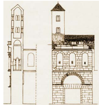
Rekonstrukcija presjeka i južnog pročelja crkve Sv. Martina
