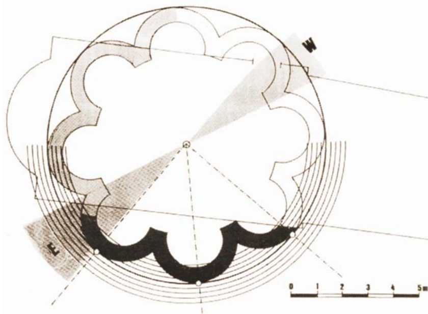
Geometrijski prikaz osmerokutne crkve ispod crkve Sv. Joakima i Ane
