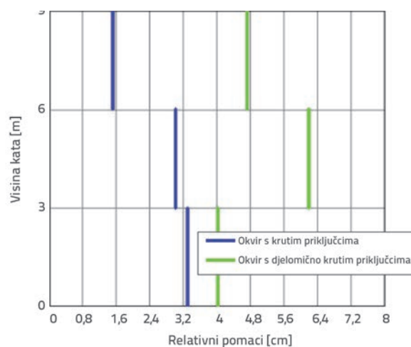
Slika 17. Prikaz apsolutnih i relativnih pomaka okvira
