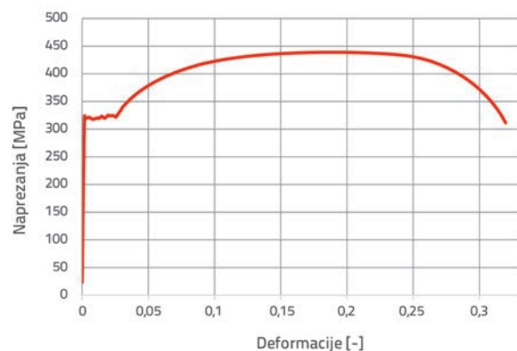
Slika 2. Materijalne karakteristike čelika za stup i gredu
