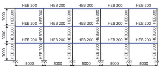
Slika 11. Geometrijske karakteristike ravninskog okvira s prikazom poprečnih presjeka
