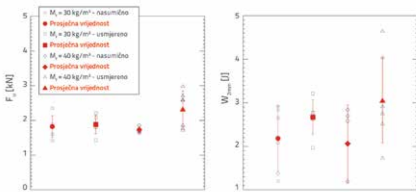
Slika 14. Granične sile F_u i disipacija energije W_{2mm} koje uzrokuju progib od 2 mm na sredini raspona za oba volumna udjela vlakana u uzorku i obje vrste orijentacije vlakana
