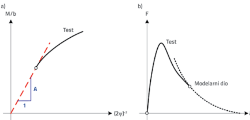
Slika 9. Shematski prikaz: a) M/b u odnosu na (2\Psi)^2 krivulju; b) modelirani dio do nulte sile
