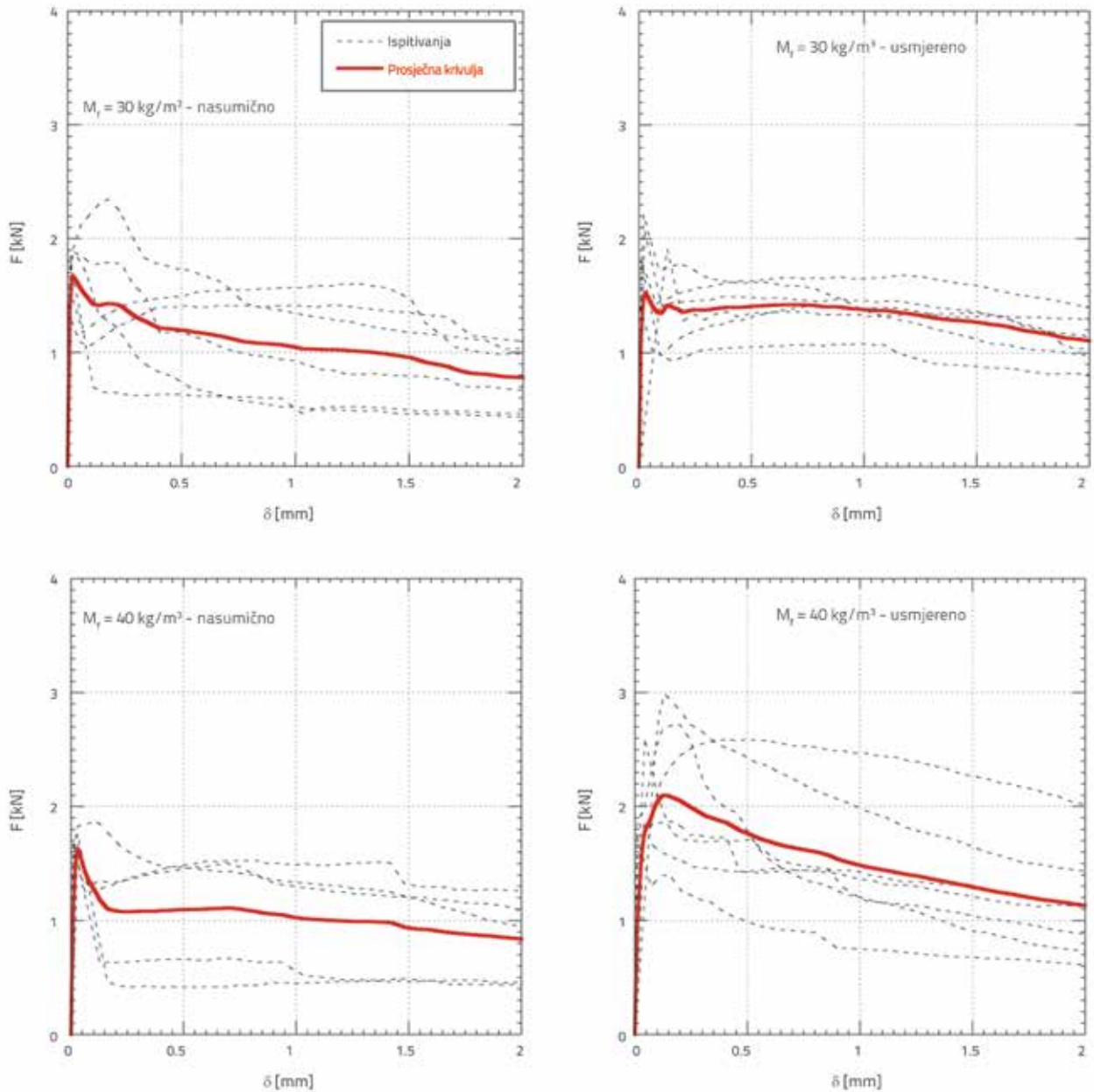
Slika 13. Krivulje "sila - progib" na sredini raspona za oba volumna udjela vlakana u uzorku i za obje vrste orijentacije vlakana
