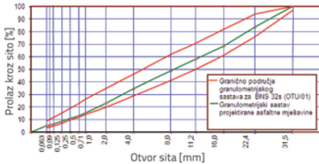
b) Ostvareni granulometrijski sastav asfaltna mješavine
