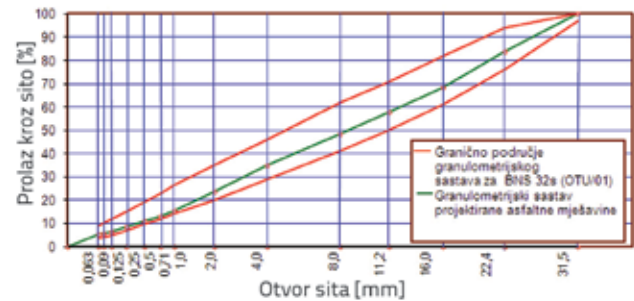
b) Ostvareni granulometrijski sastav asfaltna mješavine
