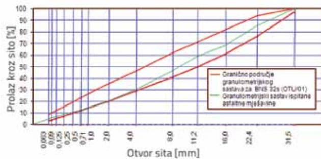
Slika 3. Granulometrijski sastav asfaltna mješavine s 25% recikliranog asfalta
